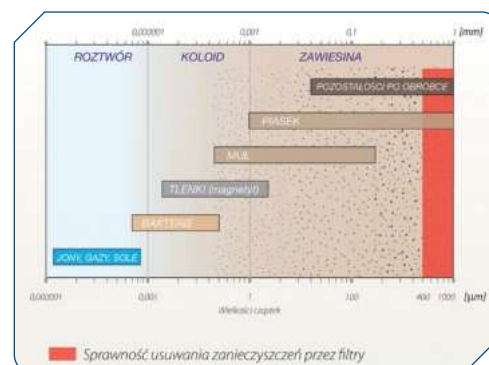
Rys. 1. Sprawność usuwania zanieczyszczeń przez filtry
