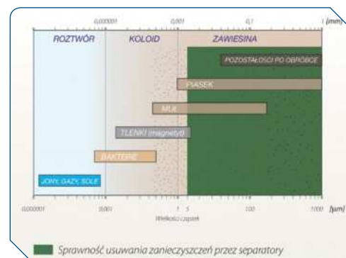
Rys. 2. Sprawność usuwania zanieczyszczeń przez separator
